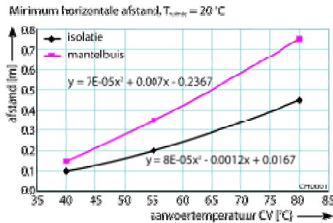
Figuur 12. Interpolatie bij andere cv-aanvoertemperaturen
