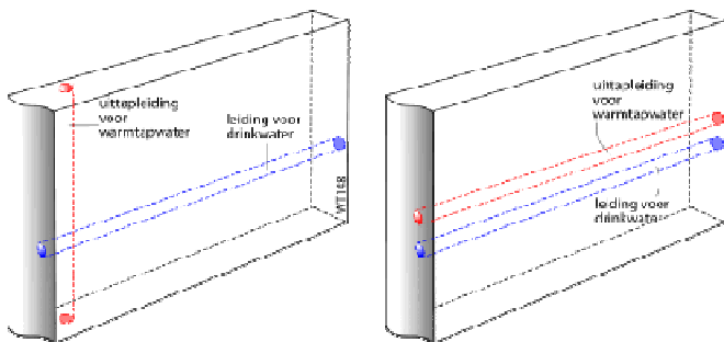
Figuur 16. Leiding voor drinkwater of huishoudwater kruist uittapleiding warmtapwater, of loopt parallel daaraan in de wand of vloer (toegestaan)
