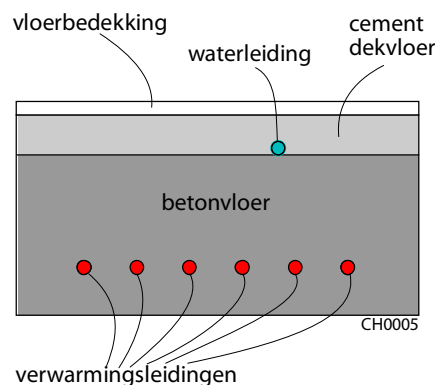
Figuur 24. Waterleiding in cement dekvloer op een vloer met betonkernactivering (28 °C).
