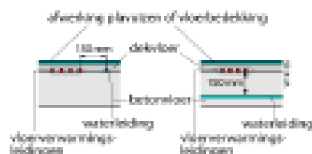
Figuur 19. Minimumafstanden van voorbeeld 5.
