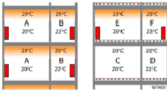
Figuur 9. Temperaturen en temperatuurgelaagdheid in ruimten met radiator- en met vloerverwarming (De coderingen A t/m F worden toegepast in tabellen 2, 4 en 5)
