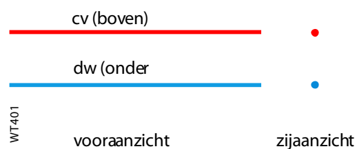
Figuur 1. Waterleiding parallel aan warme leiding (opbouw)
