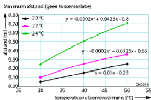
Figuur 20. Interpolatie bij andere aanvoertemperaturen vloerverwarming
